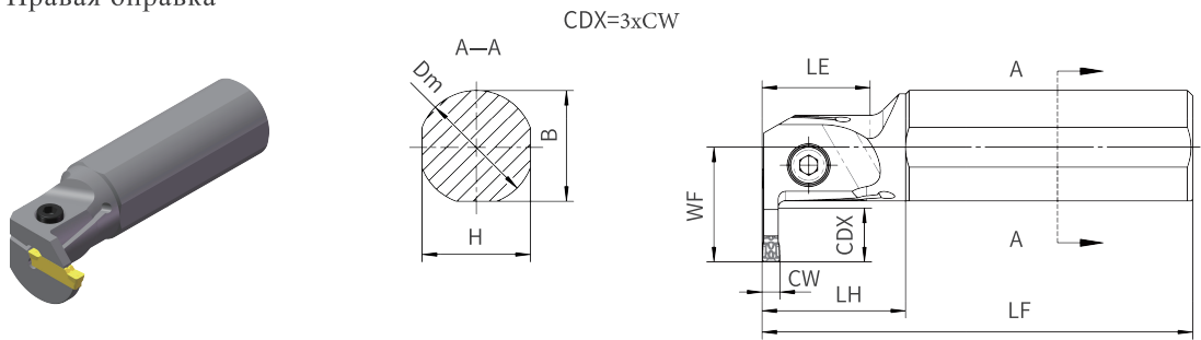
Правая оправка
