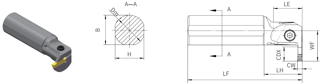
Левая оправка
