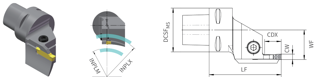
Левая головка
