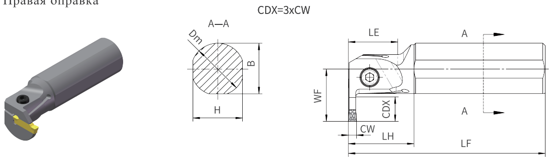
Правая оправка
